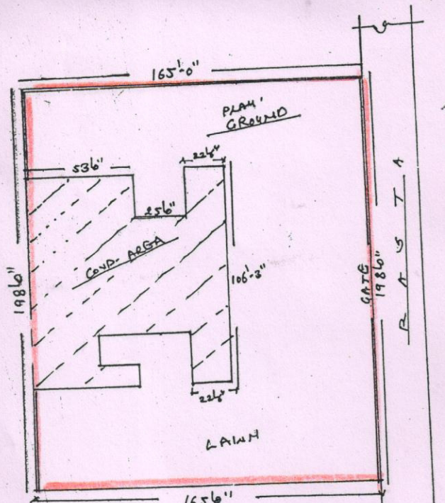
SITE PLAN (1:320)
